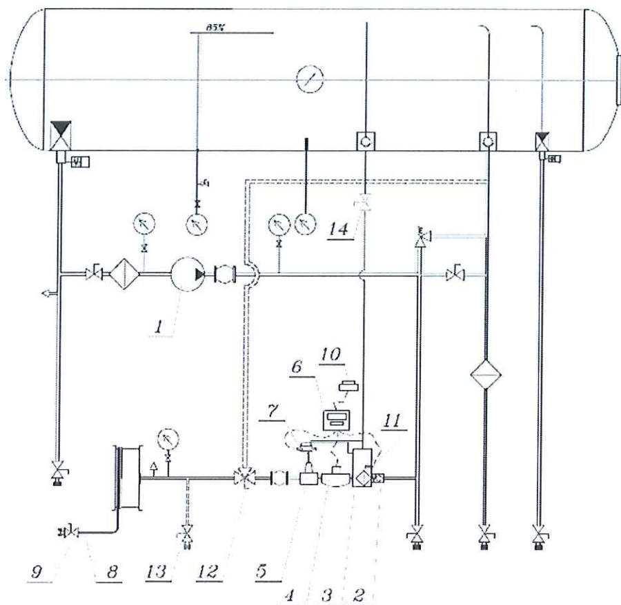
Rysunek nr 1: Schemat instalacji pomiarowej IPM-01-xx zamontowanej na cysternie drogowej
